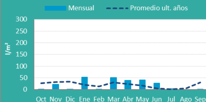
Precipitación media mensual-Sistema IV
