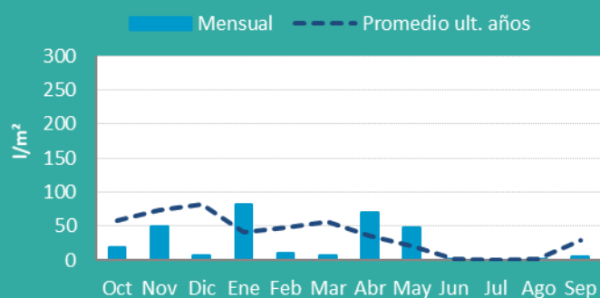
Precipitación media mensual-Subsistema 14
