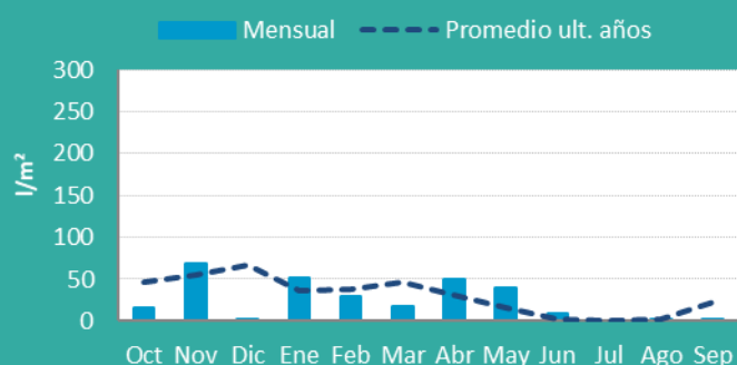
Precipitación media mensual-Sistema III
