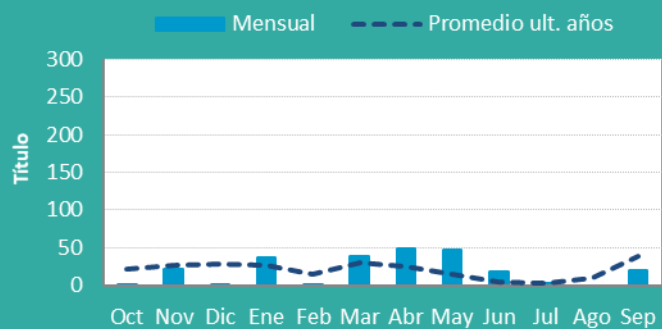
Precipitación media mensual-Sistema V
